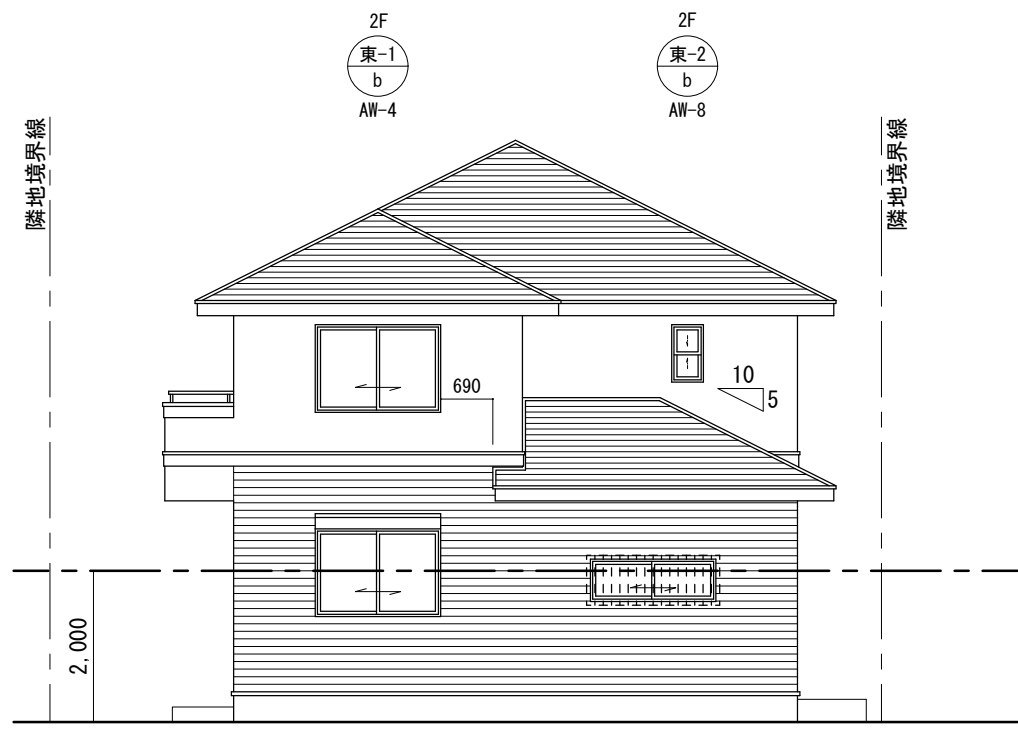
東立面図 S:1/100
